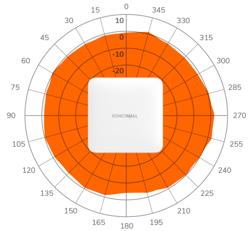
2.4GHz, XZ-Plane
