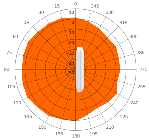
5GHz, XY-Plane
